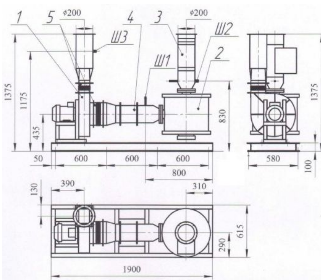
Типовая компоновка УСЖ
